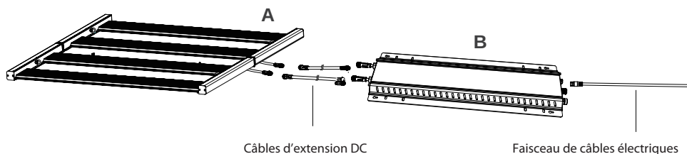
Câbles d'extension DC
